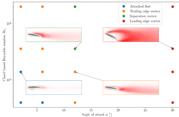
Régimes d'écoulement en fonction du nombre de Reynolds et de l'angle d'attaque
